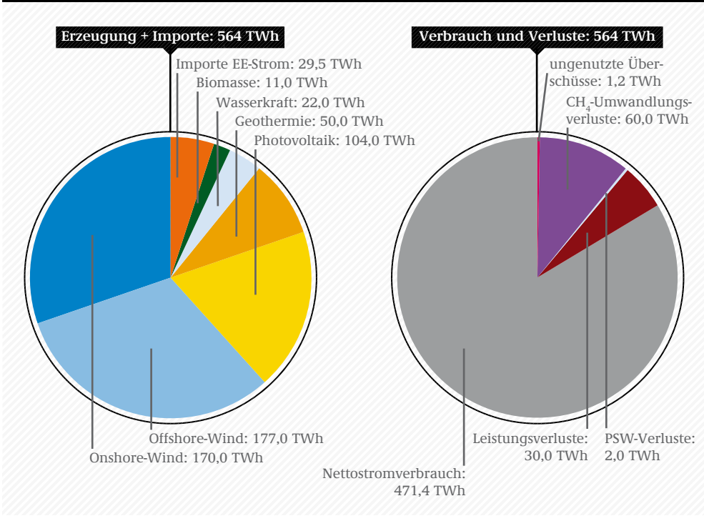
ABB 7-26 NETTOSTROMERZEUGUNG OHNE SPEICHERKRAFTWERKE ZUZÜGLICH IMPORTE AUS ERNEUERBAREN ENERGIEN SOWIE NETTOSTROMVERBRAUCH UND VERLUSTE ALS MITTELWERTE FÜR DIE WETTERJAHRE 2006-2009 FÜR DAS ERZEUGUNGSSYSTEM MIT METHANSPEICHER
