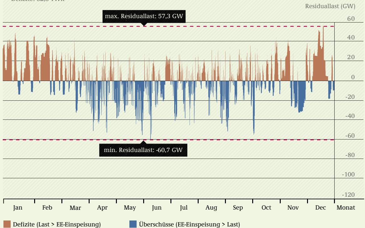
Residuallast mit allen Verbrauchern und Lastmanagement, nach PSW (Meteo-Jahr 2009)
