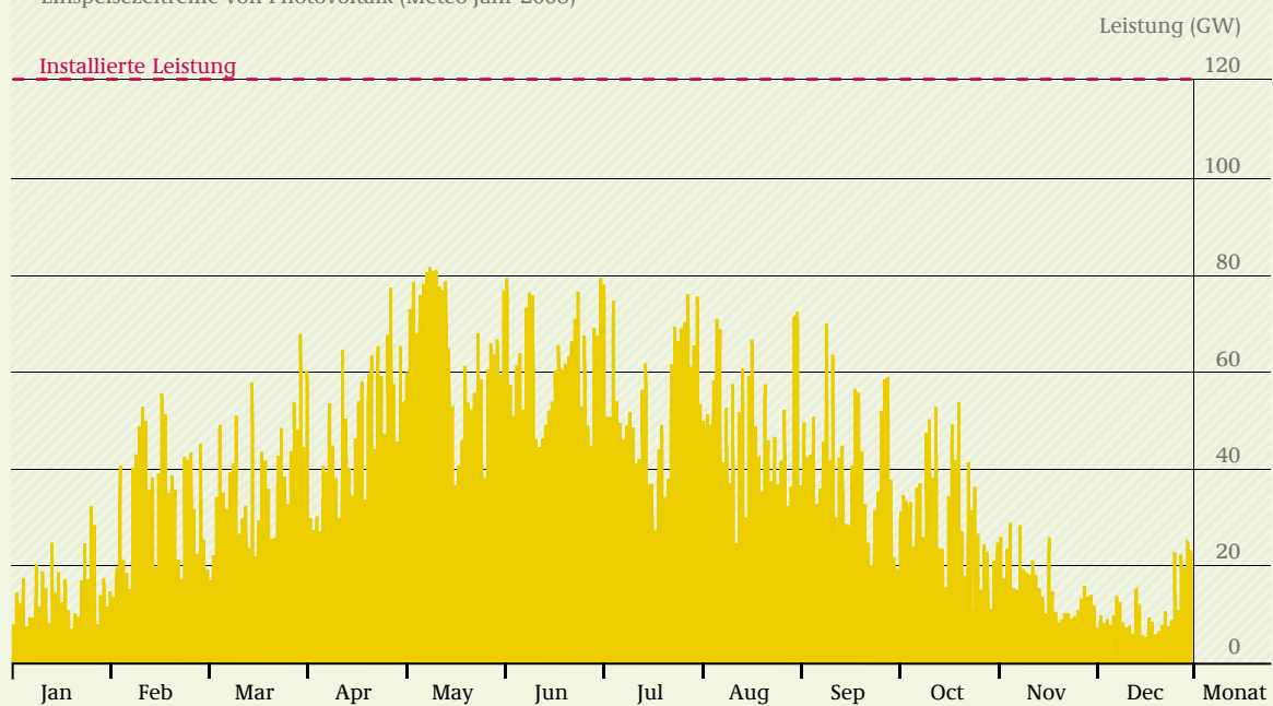
Einspeisezeitreihe von Photovoltaik (Meteo-Jahr 2008)
