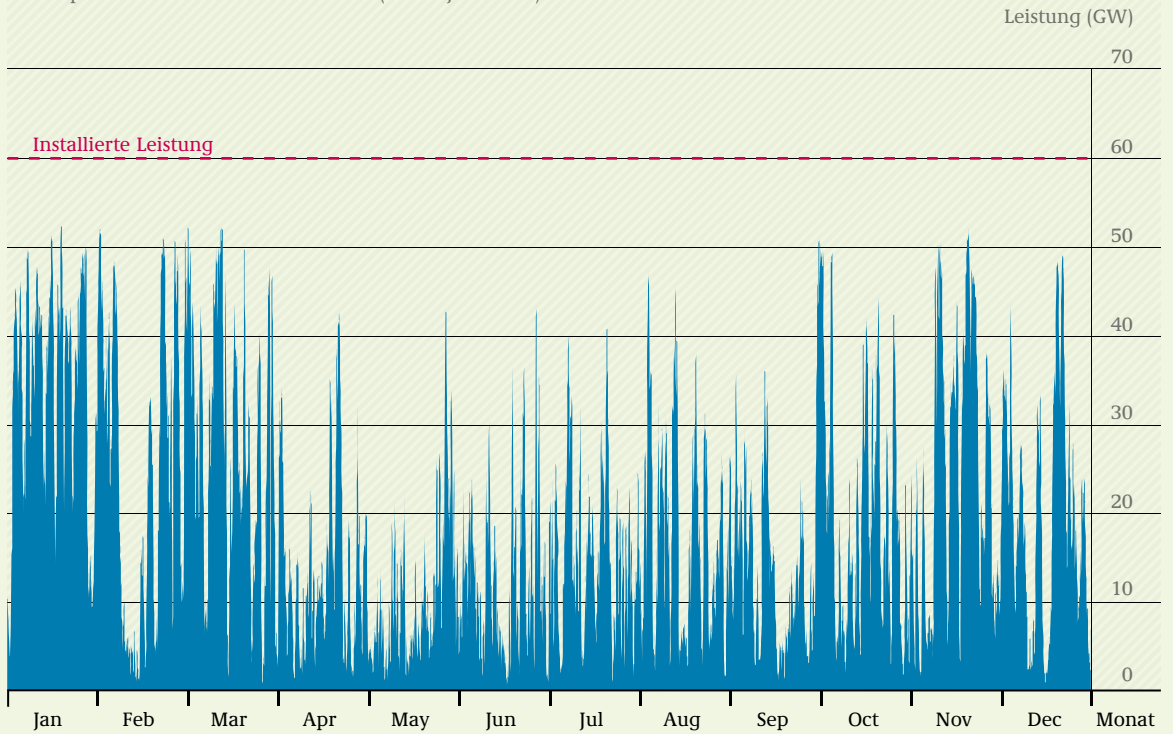
Einspeisezeitreihe von Onshore-Wind (Meteo-Jahr 2008)
