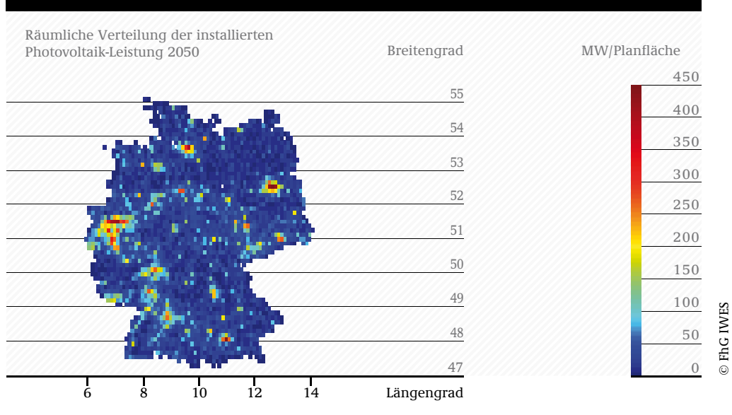
ABB 7-2 RÄUMLICHE VERTEILUNG DER PHOTOVOLTAIK
