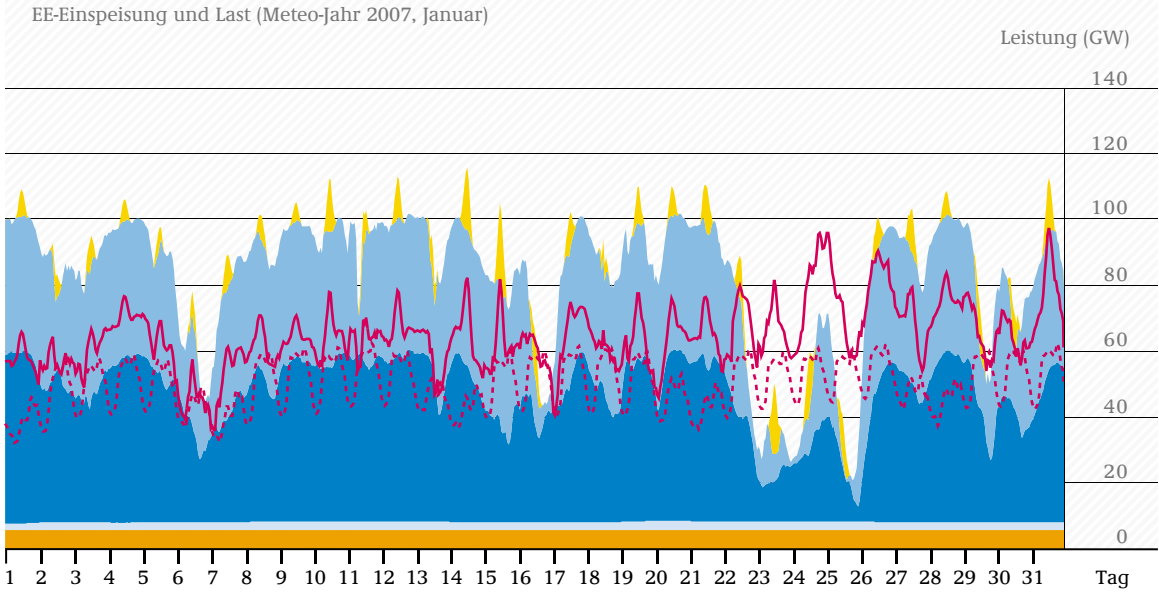
ABB 7-10 BEISPIELE FÜR DIE EINSPEISUNG DER ERNEUERBAREN ENERGIEN IM JAHR 2050, BASIEREND AUF DEM WETTER JAHR 2007 – JANUAR (OBEN), DEZEMBER (MITTE), AUGUST (UNTEN)
