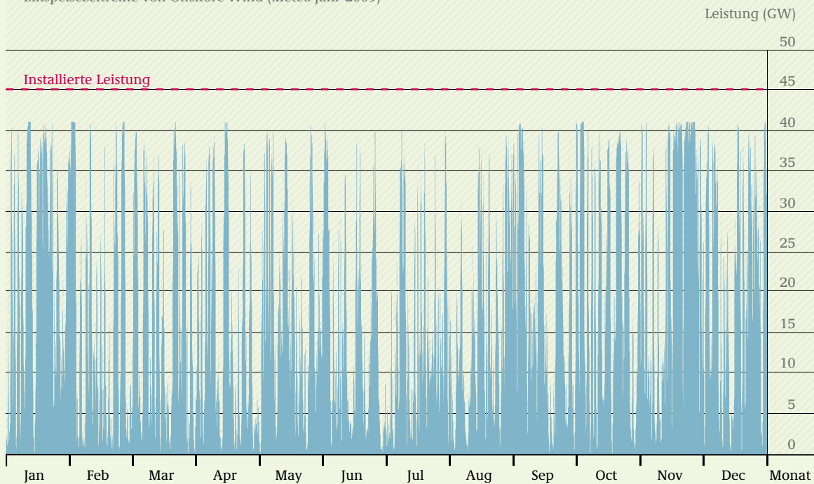
Einspeisezeitreihe von Offshore-Wind (Meteo-Jahr 2009)
