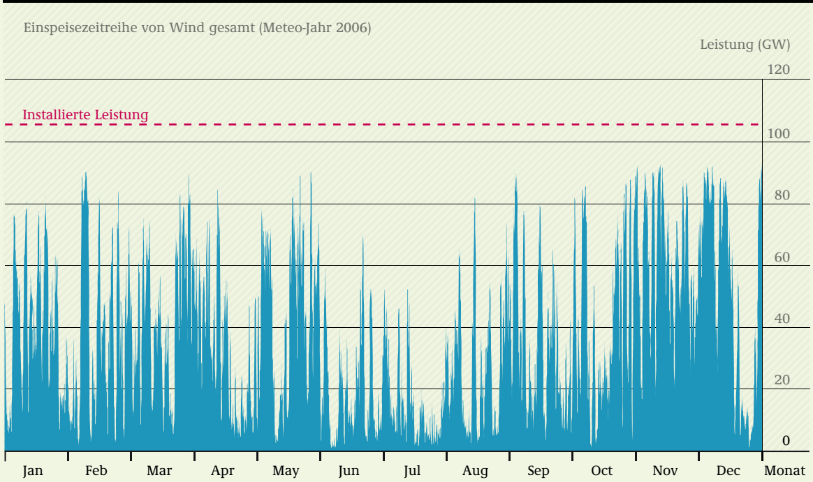
ABB 10-4 MITTLERE STÜNDLICHE EINSPEISUNG WIND GESAMT (ONSHORE UND OFFSHORE) IM JAHR 2050, FÜR ALLE WETTER-JAHRE 2006-2009
