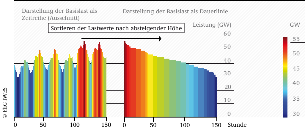
ABB 7-14 BEISPIELHAFTER AUFBAU UND ABLEITUNG EINER JAHRESDAUERLINIE (HIER: EINER WOCHE)
