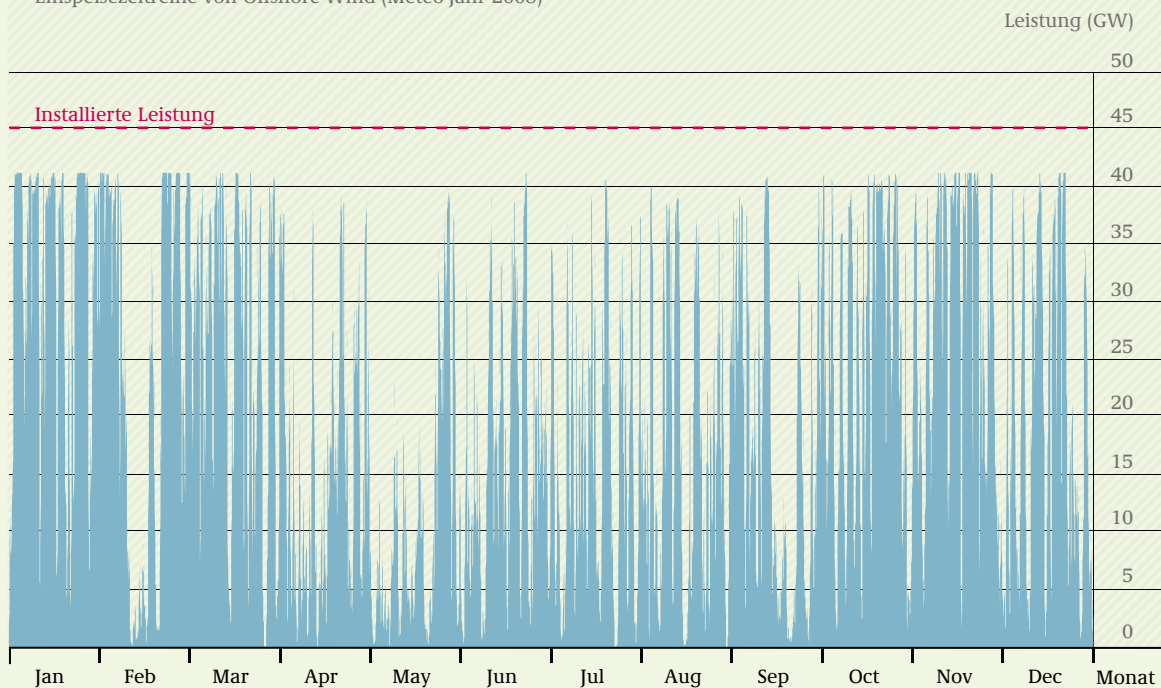
Einspeisezeitreihe von Offshore-Wind (Meteo-Jahr 2008)
