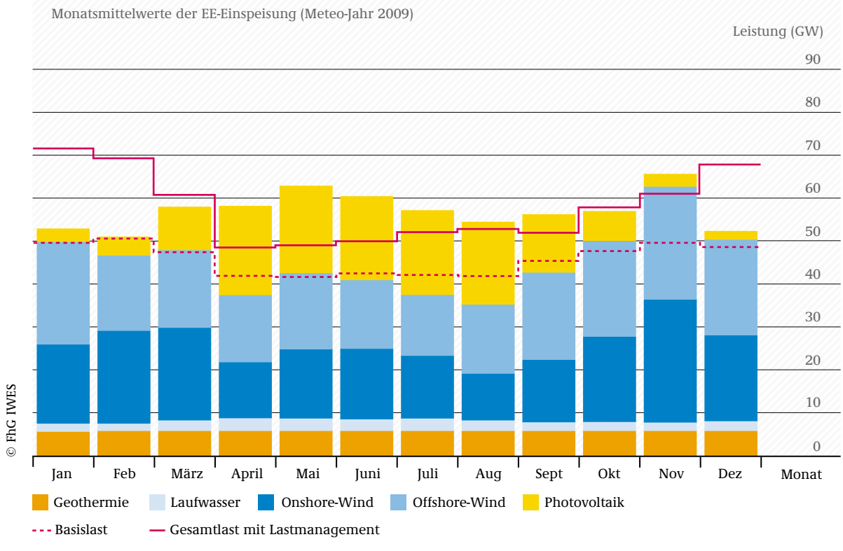
ABB 7-9 MONATLICHE EINSPEISUNG ALLER ERNEUERBARER ENERGIEN, INKL. DARSTELLUNG DER LAST VOR UND NACH DEM LASTMANAGEMENT IM JAHR 2050, BEISPIELHAFT BASIEREND AUF DEM WETTER-JAHR 2009, DARSTELLUNG ALS MONATLICHE MITTELWERTE 200
