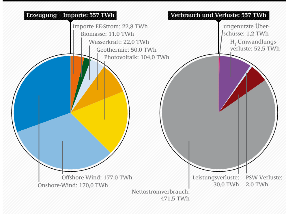
ABB 7-25 NETTOSTROMERZEUGUNG OHNE SPEICHERKRAFTWERKE ZUZÜGLICH IMPORTE AUS ERNEUERBAREN ENERGIEN SOWIE NETTOSTROMVERBRAUCH UND VERLUSTE ALS MITTELWERTE FÜR DIE WETTERJAHRE 2006-2009 FÜR DAS ERZEUGUNGSSYSTEM MIT WASSERSTOFFSPEICHER
