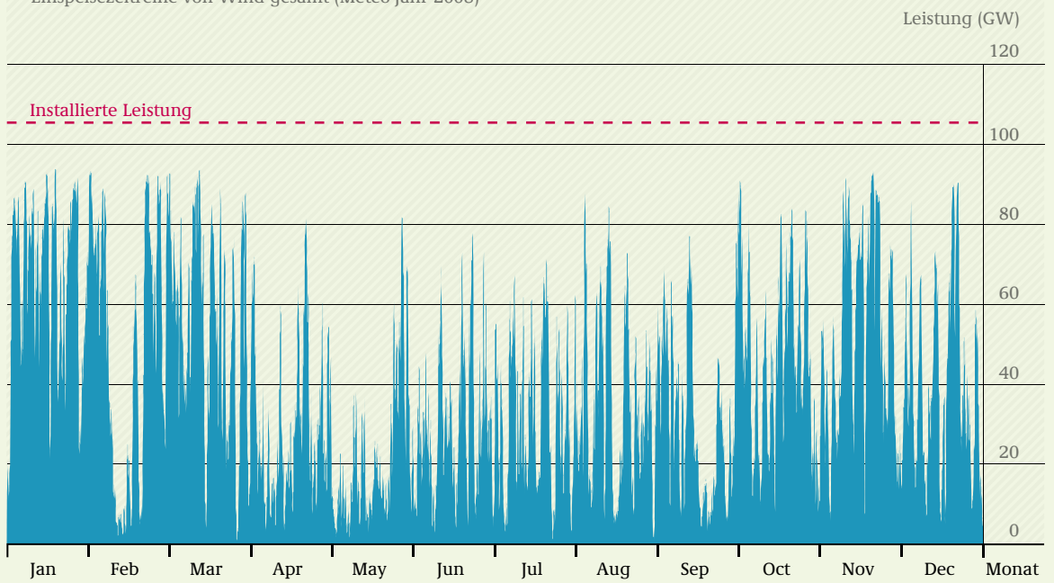
Einspeiszeitreihe von Wind gesamt (Meteo-Jahr 2008)
