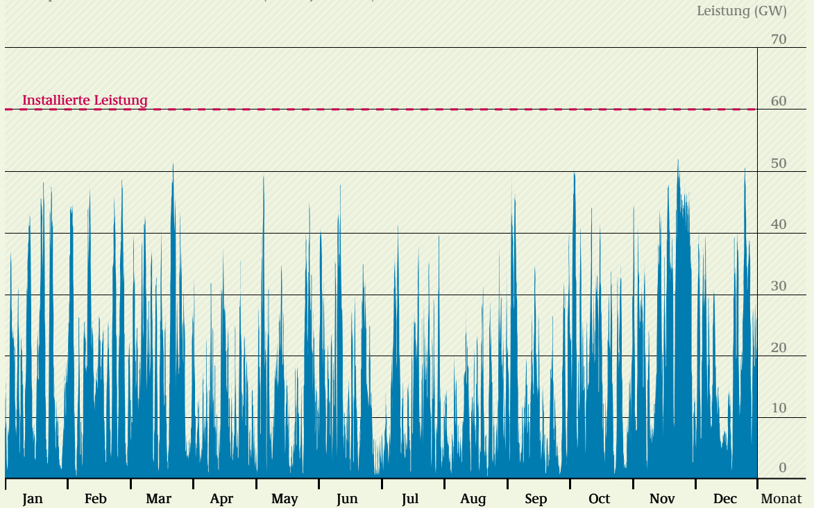
Einspeisezeitreihe von Onshore-Wind (Meteo-Jahr 2009)
