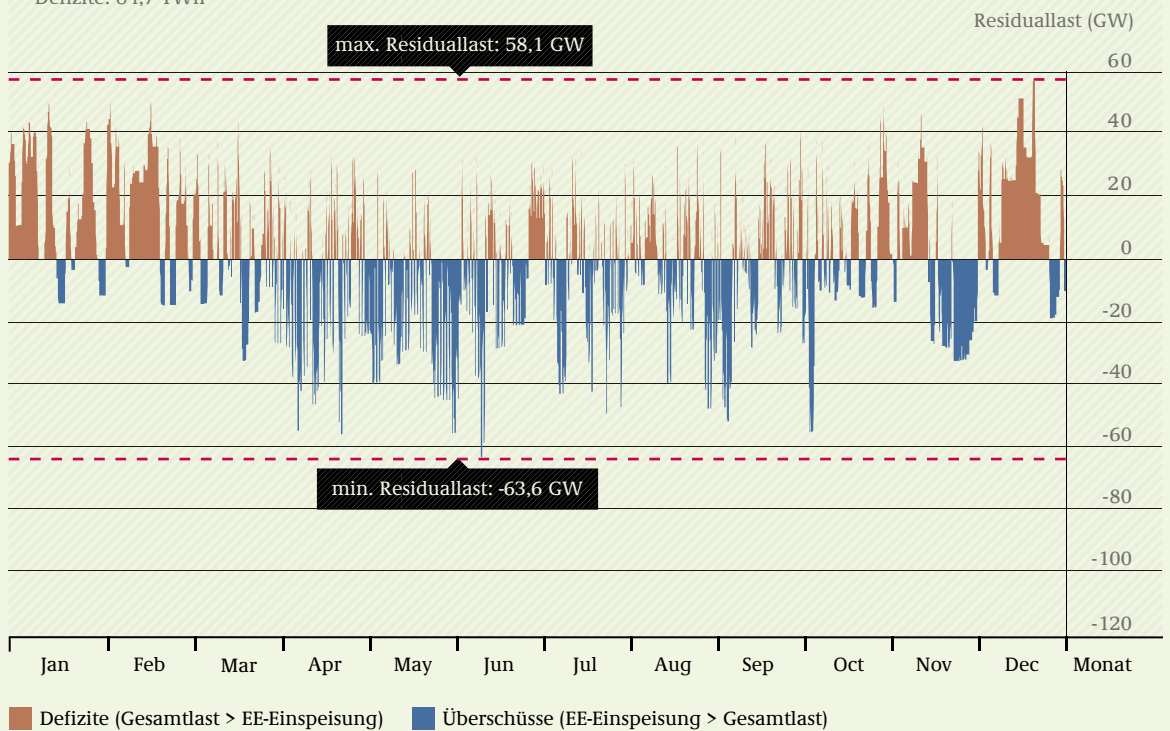
Residuallast mit allen Verbrauchern und Lastmanagement, vor PSW (Meteo-Jahr 2009)
