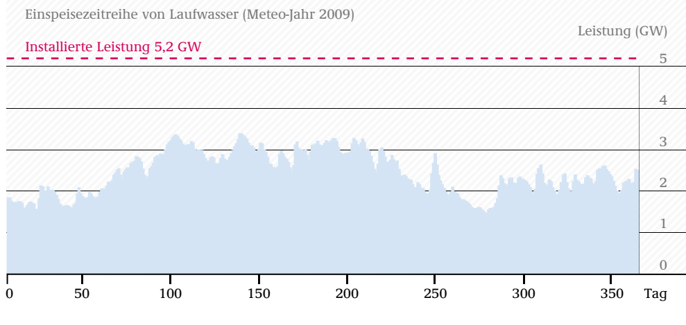
ABB 7-7 EINSPEISUNG VON WASSERKRAFT IM JAHR 2050, BASIEREND AUF DEM WETTER-JAHR 2009, DARSTELLUNG ALS TÄGLICHE MITTELWERTE
