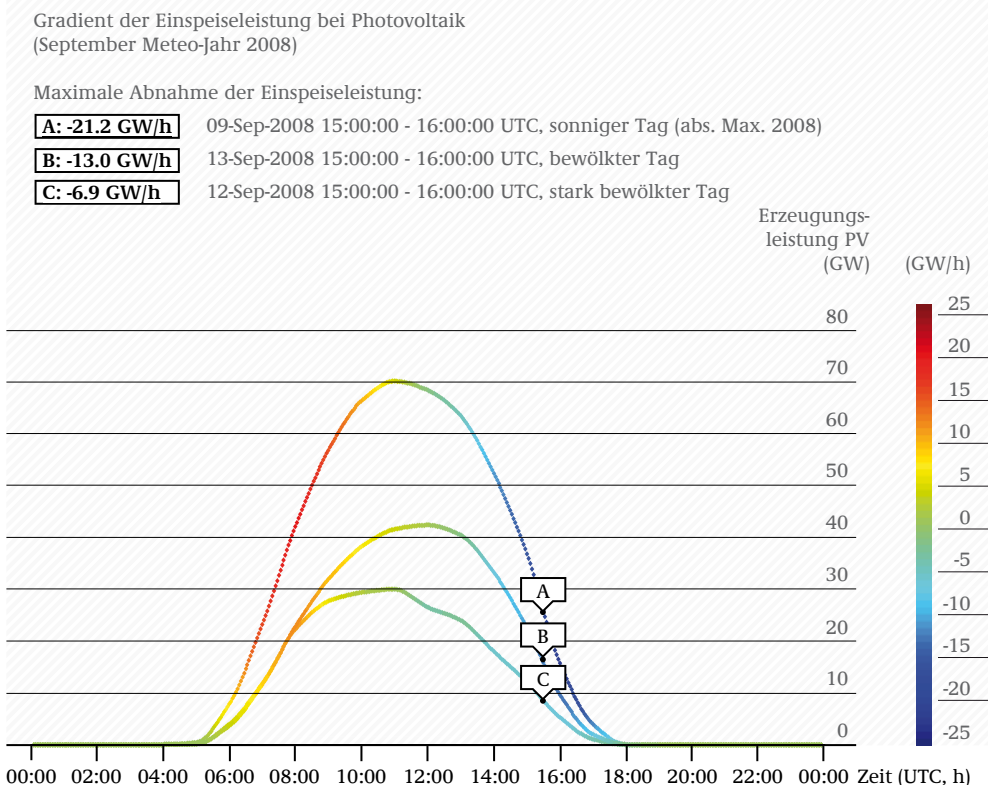
ABB 7-28 LEISTUNGSGRADIENTEN DER PV IN ABHÄNGIGKEIT VON DER MAX. TAGESLEISTUNG
