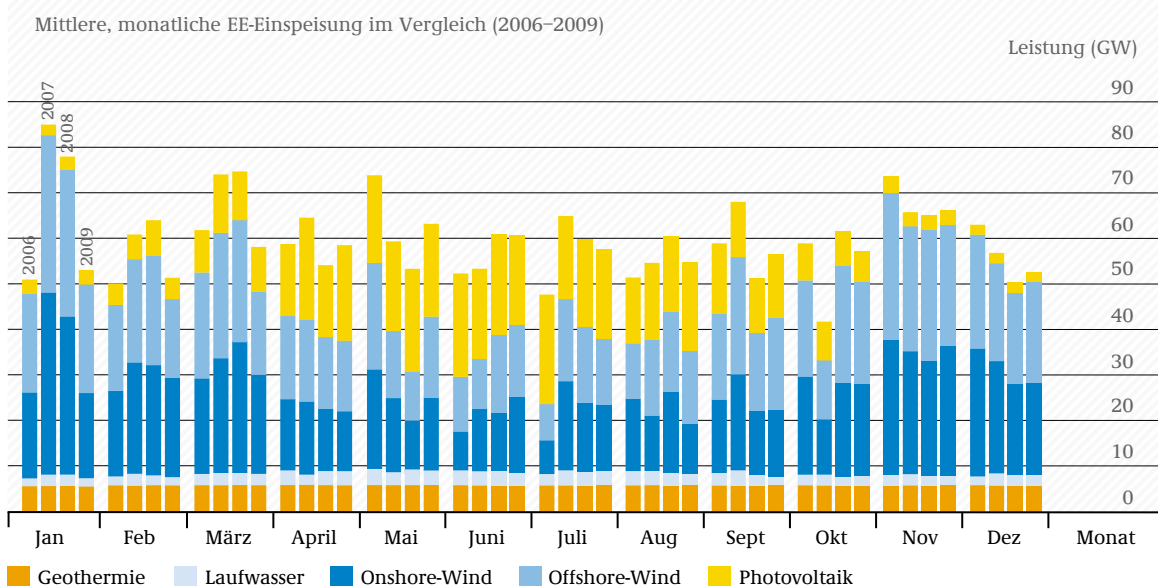
ABB 7-8 MONATLICHE EINSPEISUNG ALLER ERNEUERBARER ENERGIEN, DARGESTELLT FÜR ALLE WETTER-JAHRE 2006-2009, DARSTELLUNG ALS MONATLICHE MITTELWERTE
