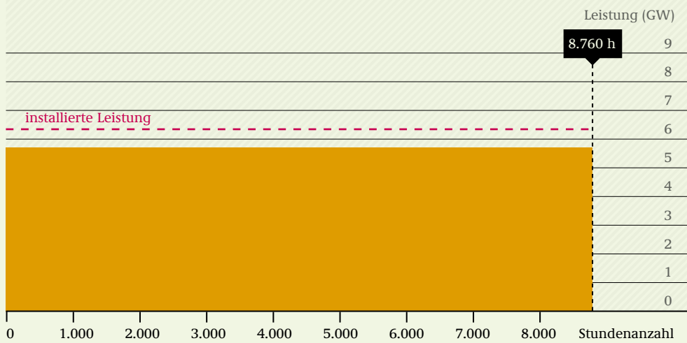
Jahresdauerlinie von Geothermie (Meteo-Jahr 2009)
