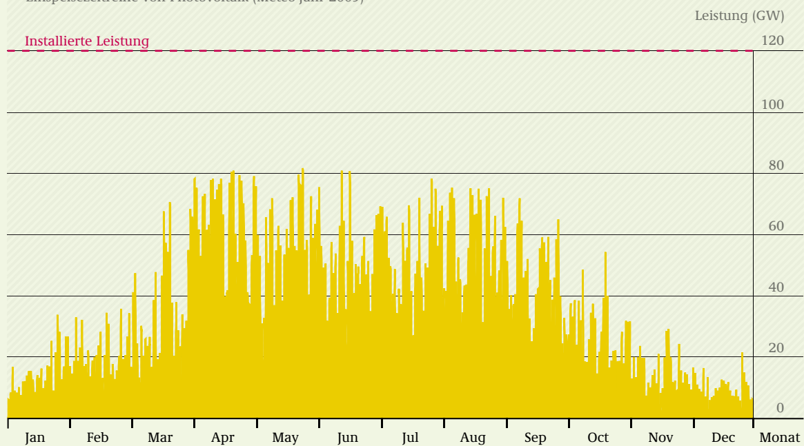
Einspeisezeitreihe von Photovoltaik (Meteo-Jahr 2009)
