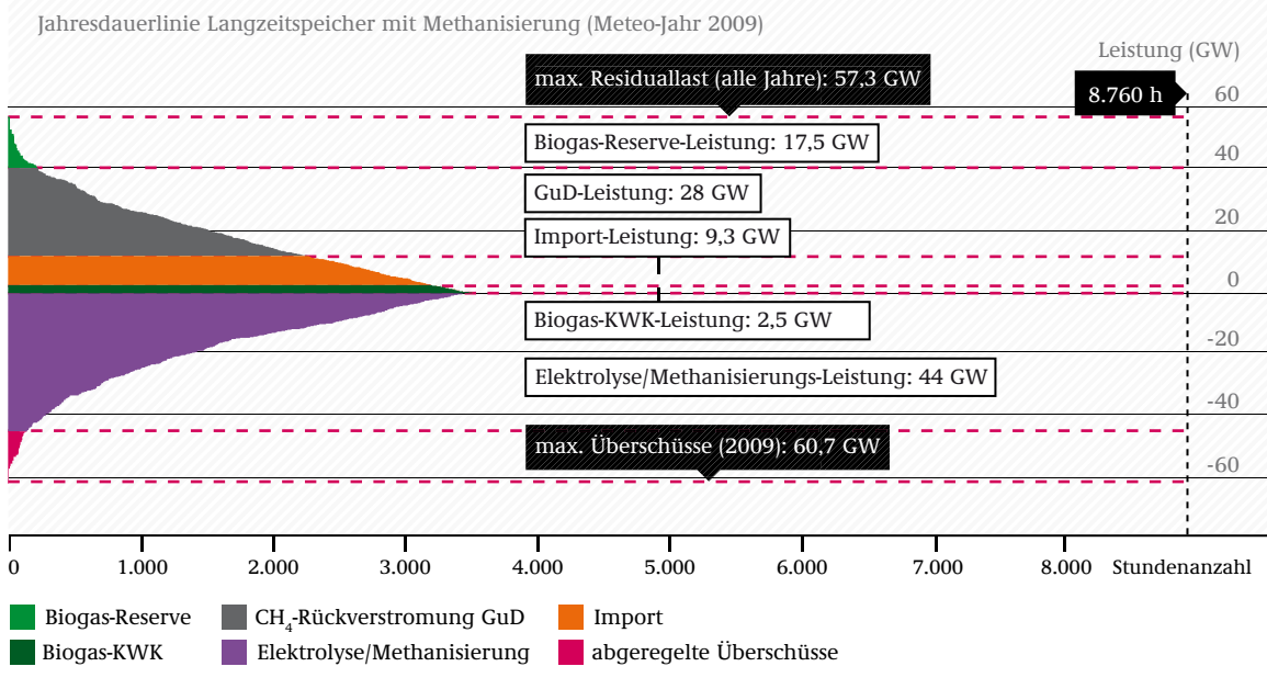
ABB 7-24 JAHRESDAUERLINIE VON ELEKTROLYSE/METHANISIERUNG, METHAN-RÜCKVERSTROMUNG, BIOGASVERSTROMUNG UND IMPORTEN IM JAHR 2050, BASIEREND AUF DEM WETTER-JAHR 2009 210
