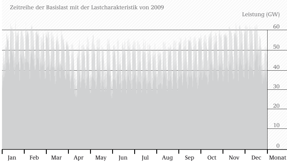
ABB 7-3 MITTLERE STÜNDLICHE BASISLAST MIT DER LASTCHARAKTERISTIK DES JAHRES 2009
