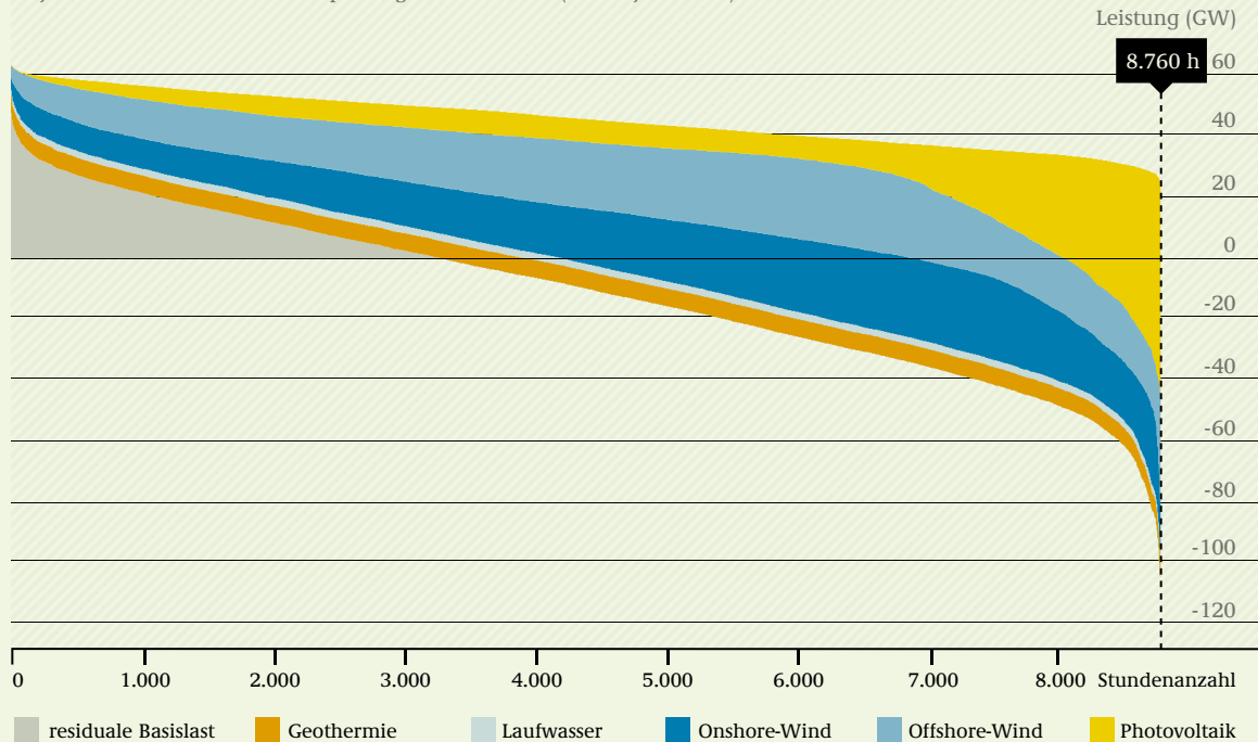
Jahresdauerlinien der EE-Einspeisung sowie der Last (Meteo-Jahr 2009)
