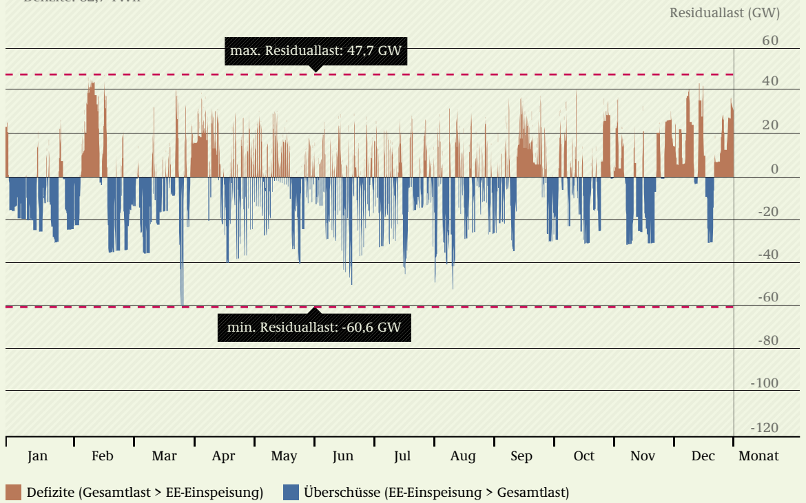
Residuallast mit allen Verbrauchern und Lastmanagement, vor PSW (Meteo-Jahr 2008)
