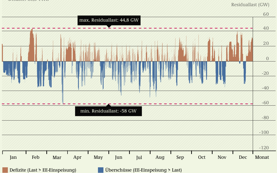
Residuallast mit allen Verbrauchern und Lastmanagement, nach PSW (Meteo-Jahr 2008)
