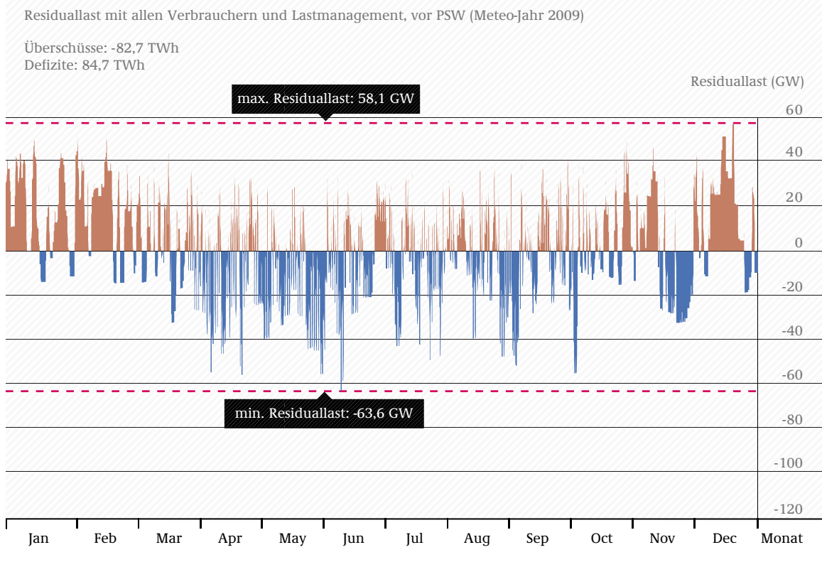
ABB 7-12 RESIDUALE GESAMTLAST (UNTER BERÜCKSICHTIGUNG VON LASTMANAGEMENT, ABER OHNE PUMPSPEICHER) FÜR DAS JAHR 2050, BASIEREND AUF DEM WETTER-JAHR 2009
