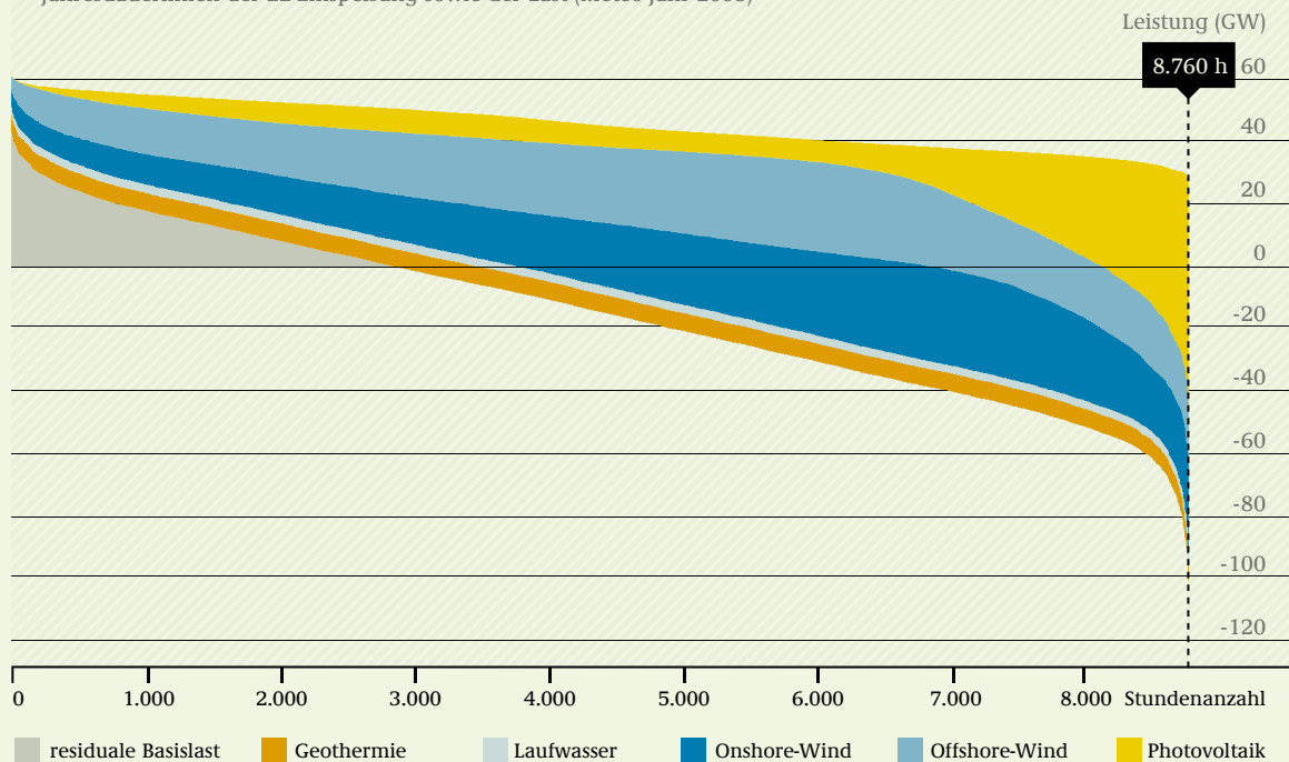
Jahresdauerlinien der EE-Einspeisung sowie der Last (Meteo-Jahr 2008)
