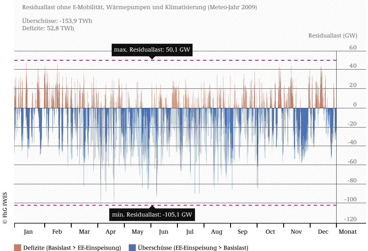
ABB 7-11 RESIDUALE BASISLAST FÜR DAS JAHR 2050, BASIEREND AUF DEM WETTER-JAHR 2009
