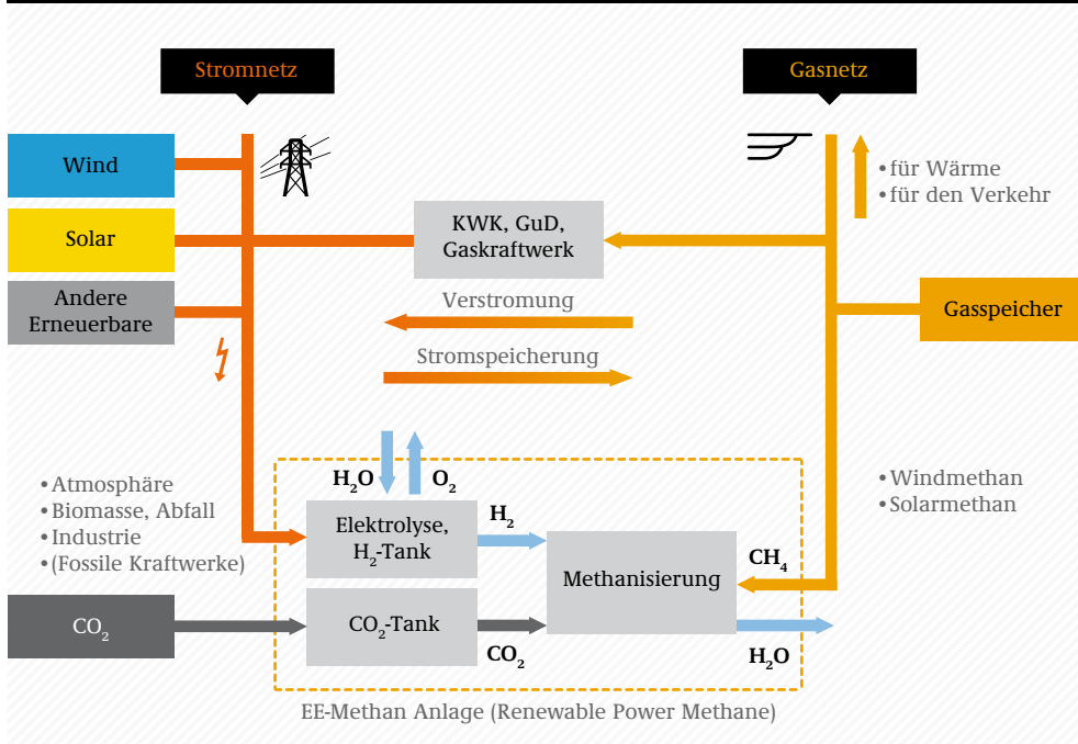
ABB 4-1 KONZEPT ZUR WANDLUNG ÜBERSCHÜSSIGEN STROMS AUS EE-ANLAGEN (WIND, PHOTOVOLTAIK) VIA WASSERSTOFF ZU METHAN (SNG) MIT RÜCKVERSTROMUNG IN GASTURBINEN- ODER GAS-UND DAMPFTURBINENKRAFTWERKEN (GuD) 85
